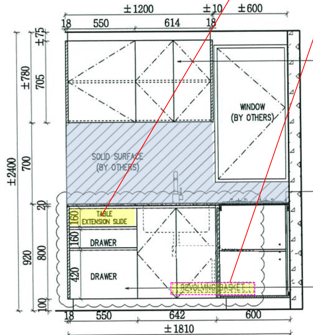
Elevation 1
