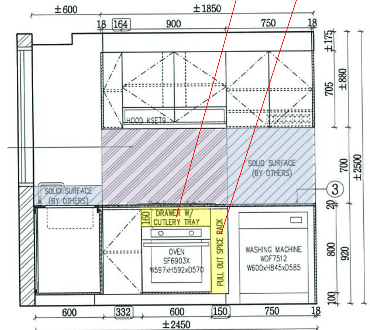
Elevation 2
